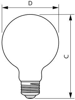
CandIG25120V2.7-25W250lm2700-2200KE26DCL
