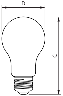
Bulb A19 120V 4.5-40W Im Green K E26 ND
