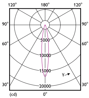
LEDspot 25,5 PAR30L 930 S15
