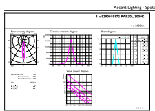
LEDspot 25,5 PAR30L 930 S15
