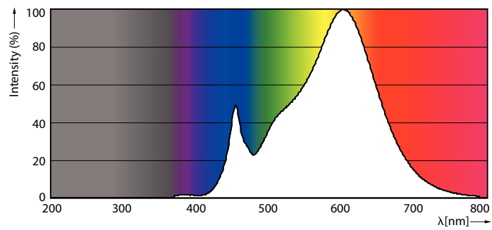
LEDspot 25,5 PAR30L 830 F25
