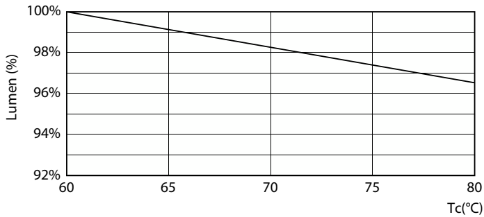
LEDtube_PLCT_8W_30K_LumenVsTc-LMP
