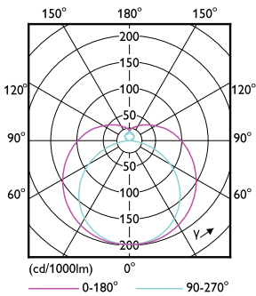
LEDtube COR NAM3 24W G5 3500lm 1-LDD
