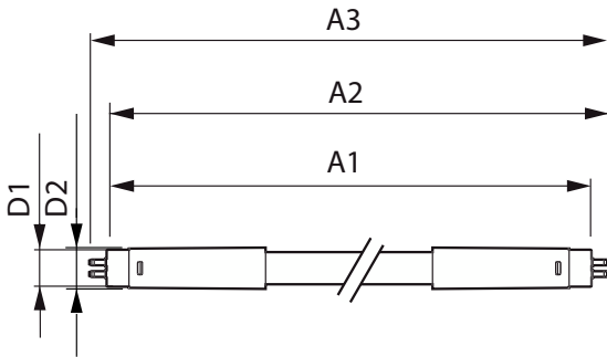
TLED T8 120-277V 14-28W 2100lm 5000K G5
