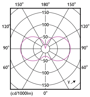
Light Distribution Diagram - 5B11/PER/CRI95WG/FR/G/E12/WGD 1CT T20
