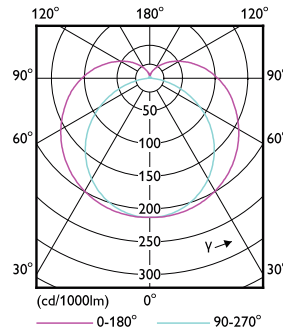
LEDtube 14W G13 2000lm
