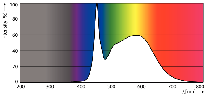
LEDtube 14W G13 2100lm 850
