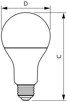
A21 29-150W 2610lm 2700-2200K E26 D
