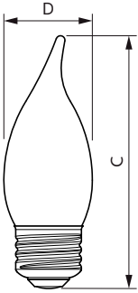
BA11 6.6-75W 600lm 2700-2200K E26 D CL
