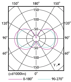
LEDbulb A15 3,3W E26 820 TA
