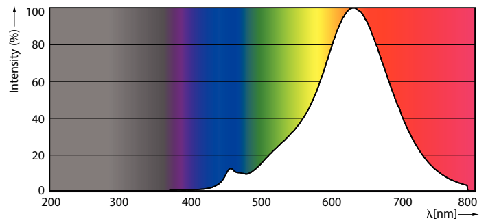
LEDbulb 3,3W A15 E26 820 TA
