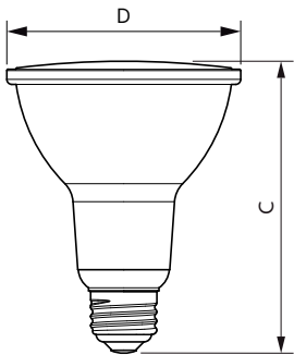
PAR30L 120V 9-75W 850lm 25D 3000K E26 D
