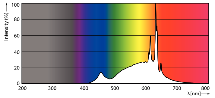
LEDbulb 12,2W A21 E26 927 FR
