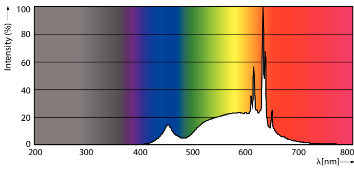
LEDspots 9,4W PAR30L E26 930 40D
