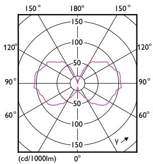
LEDbulb G16,5 4,5W E12 820 Amber
