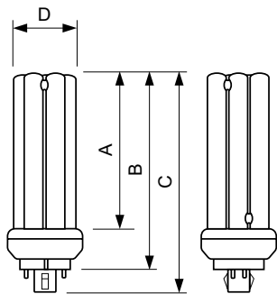
PL-T 57W/835/A/4P
