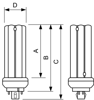
PL-T 26W/835/A/4P/ALTO
